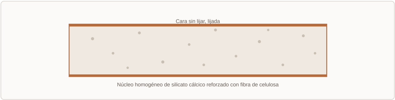
Representación esquemática de la sección de la placa; no a escala.
