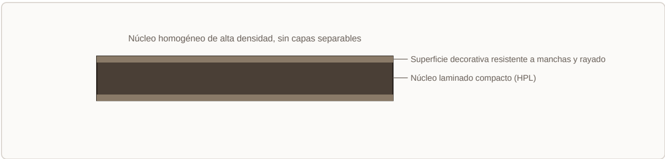
Representación esquemática de un laminado compacto homogéneo (mismo acabado y color en toda la sección); no a escala.
